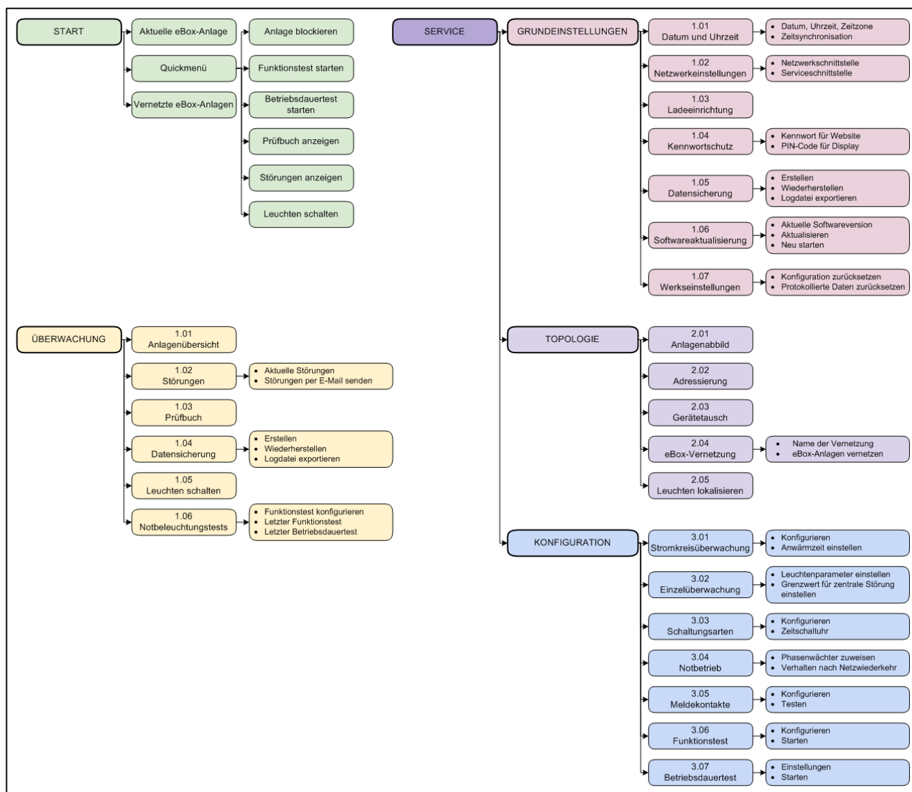
Bild 2: Menüstruktur
